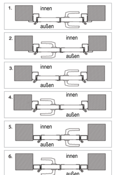
Einbauvarianten (nur Beispiel !)
