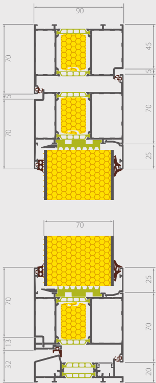
Querschnitt des Türrahmens mit einer Stärke von 90 mm samt Flügel. Füllung mit einer Stärke von 70 mm. Abbildung mit zusätzlichen Isolationseinsätzen im Flügel und Blendrahmen.
