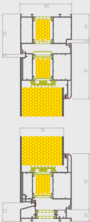
Querschnitt des Türrahmens mit einer Stärke von 90 mm samt Flügel. Füllung mit einer Stärke von 76 mm. Abbildung mit zusätzlichen Isolationseinsätzen im Flügel und Blendrahmen.
