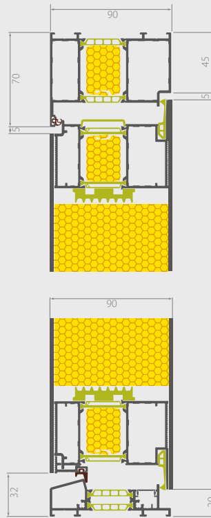
Querschnitt des Türrahmens mit einer Stärke von 90 mm samt Flügel. Füllung mit einer Stärke von 90 mm. Abbildung mit zusätzlichen Isolationseinsätzen im Flügel und Blendrahmen.
